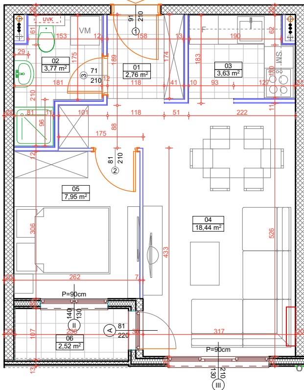
stan 38 39,07 m 2
