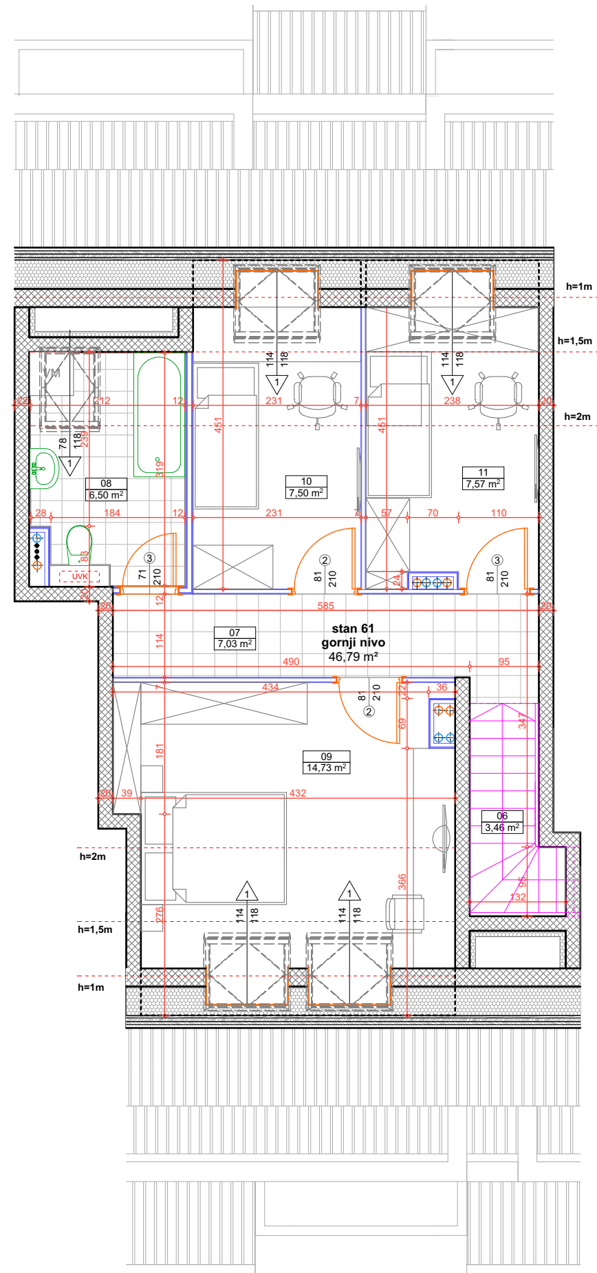
stan 61 - gornji nivo
