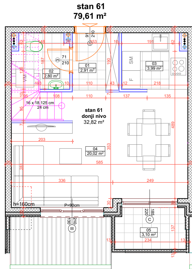
stan 61 - donji nivo
