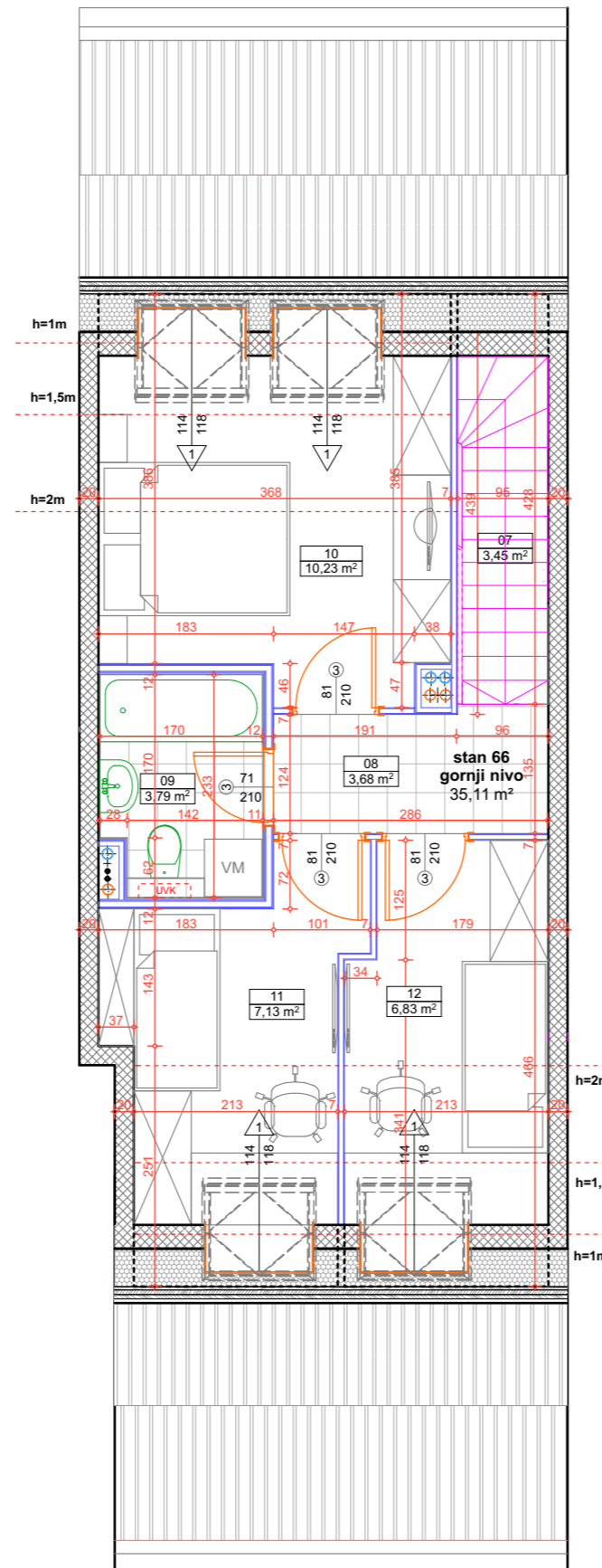
stan 66 - gornji nivo
