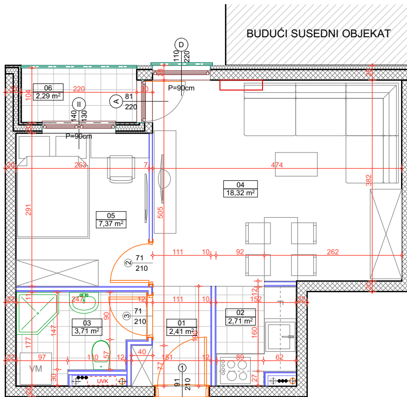
stan 55 36,81 m 2
